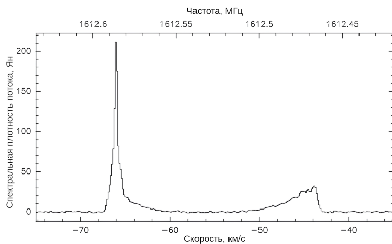
(а) Спектр области мазерного излучения.
