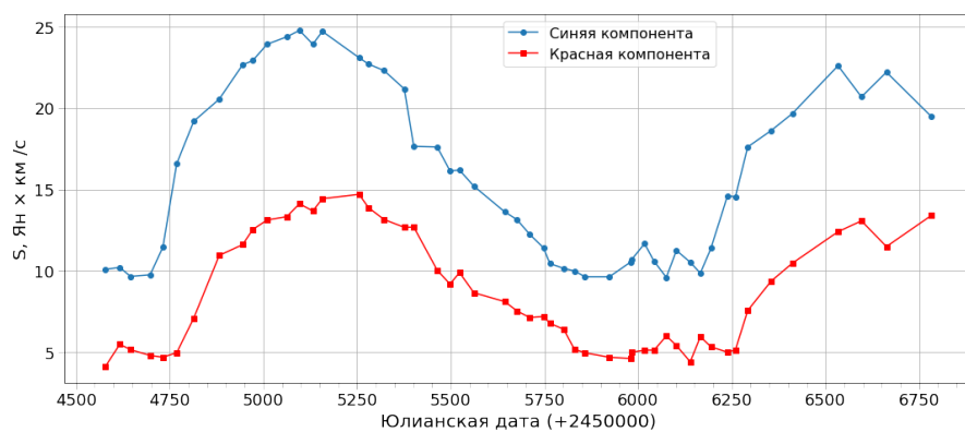
(б) Кривая блеска мазерного излучения
