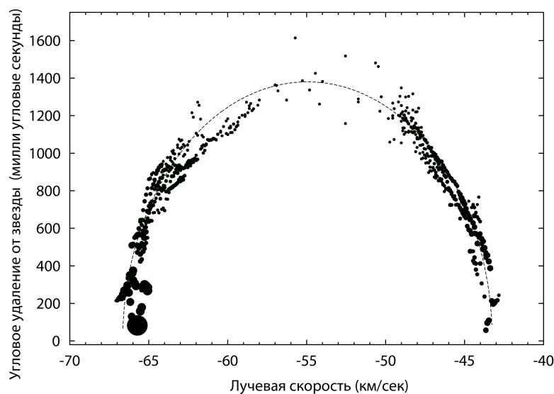
(в) Зависимость углового расстояния от звезды отдельных мазеров от их лучевых скоростей.
