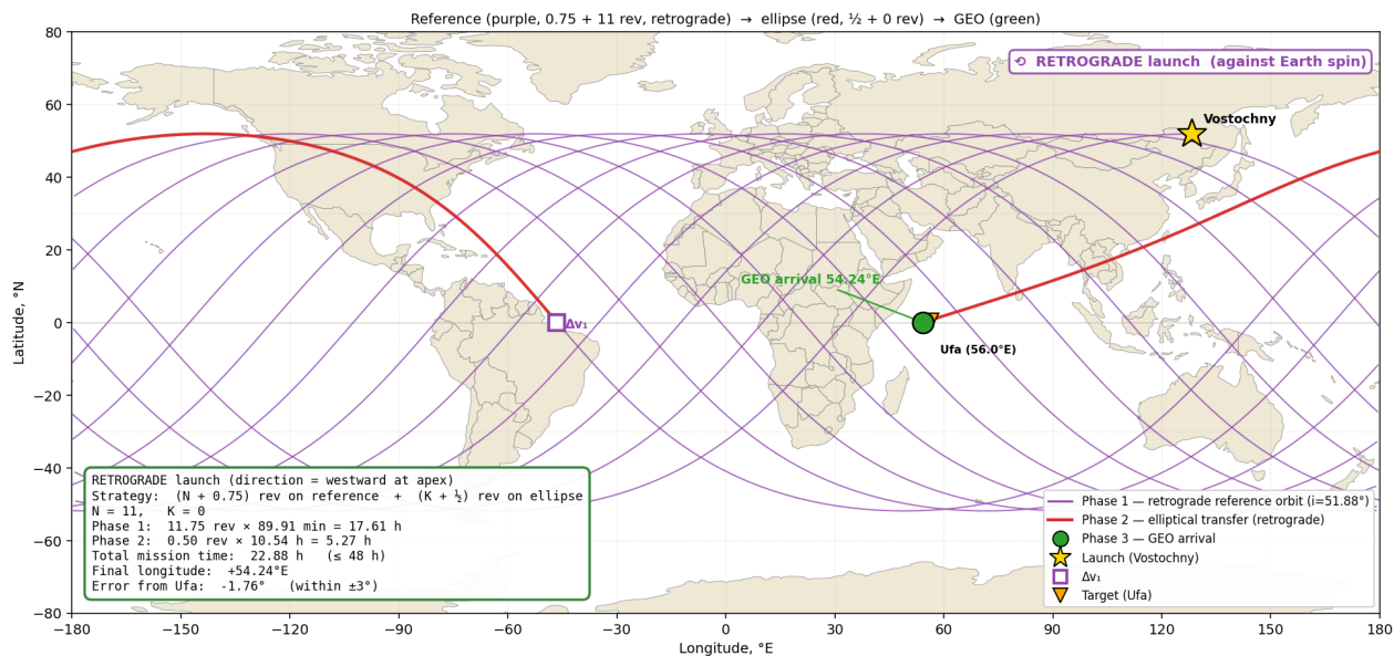
Рис. 6: Решение №2. Ретроградный запуск, n = 11 , k = 0 . \Delta T \approx 22.9 ч, конечная долгота 54.2° в. д.
