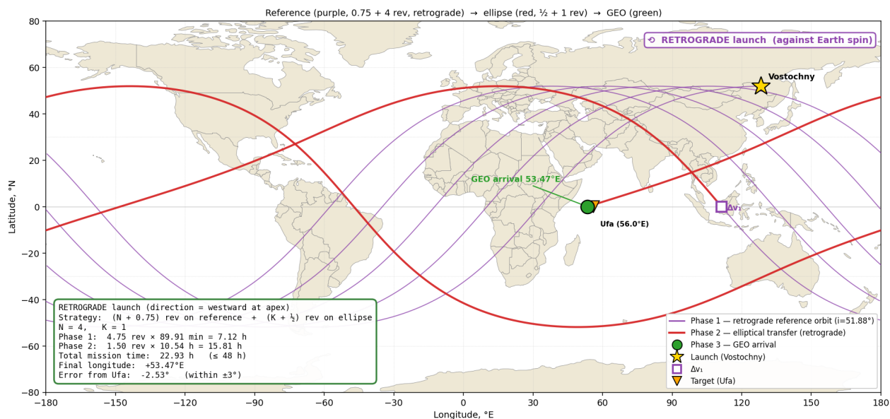
Рис. 7: Решение №3. Ретроградный запуск, n = 4 , k = 1 . \Delta T \approx 22.9 ч, конечная долгота 53.5° в. д.
