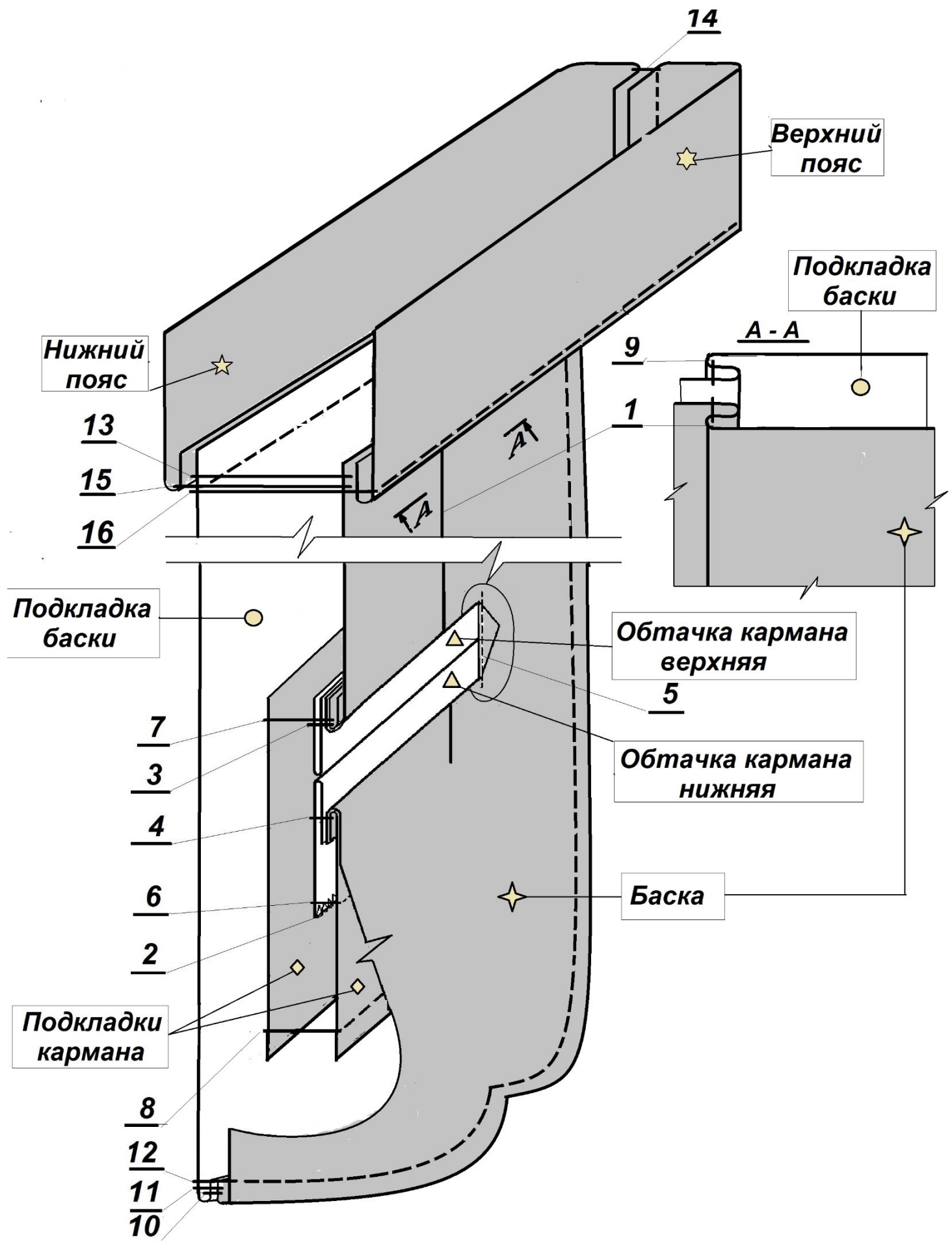
Рисунок 2 – Схема обработки баски с поясом
