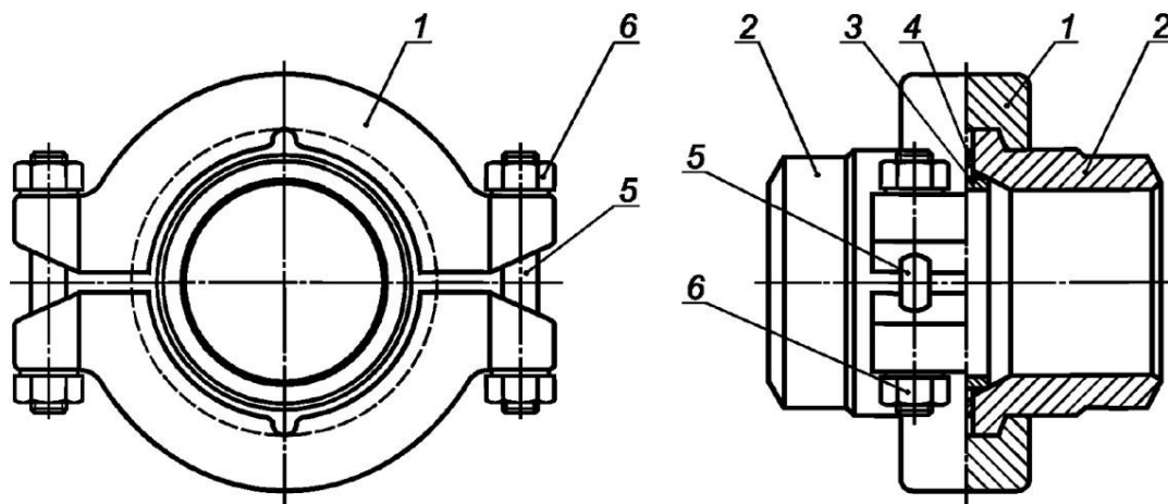
2 — ниппель; 3 — уплотнительное кольцо; 4 — упорное кольцо; 5 — шпилька по ГОСТ 10494; 6 — гайка
